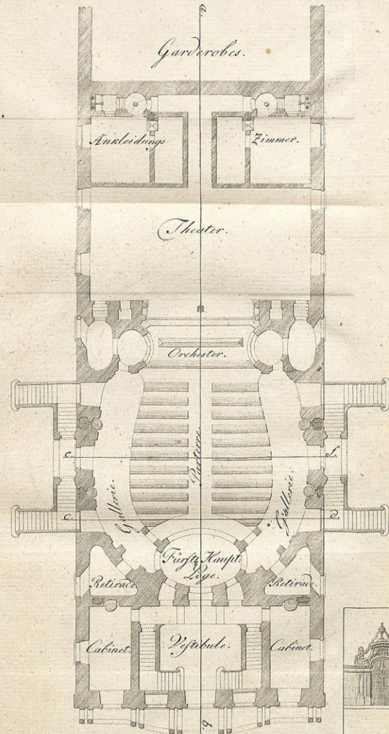
GRUNDRISS ZU EBENER ERDE.
